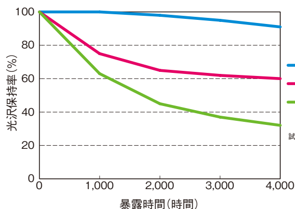
促進耐候性試験 (SWOM) 光沢保持率 (当社測定値)
